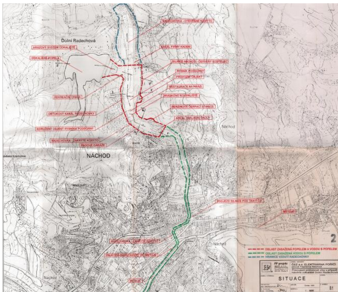
Obrázek 3: Mapa záplavového ohrožení v případě protržení hráze odkaliště Radechová
